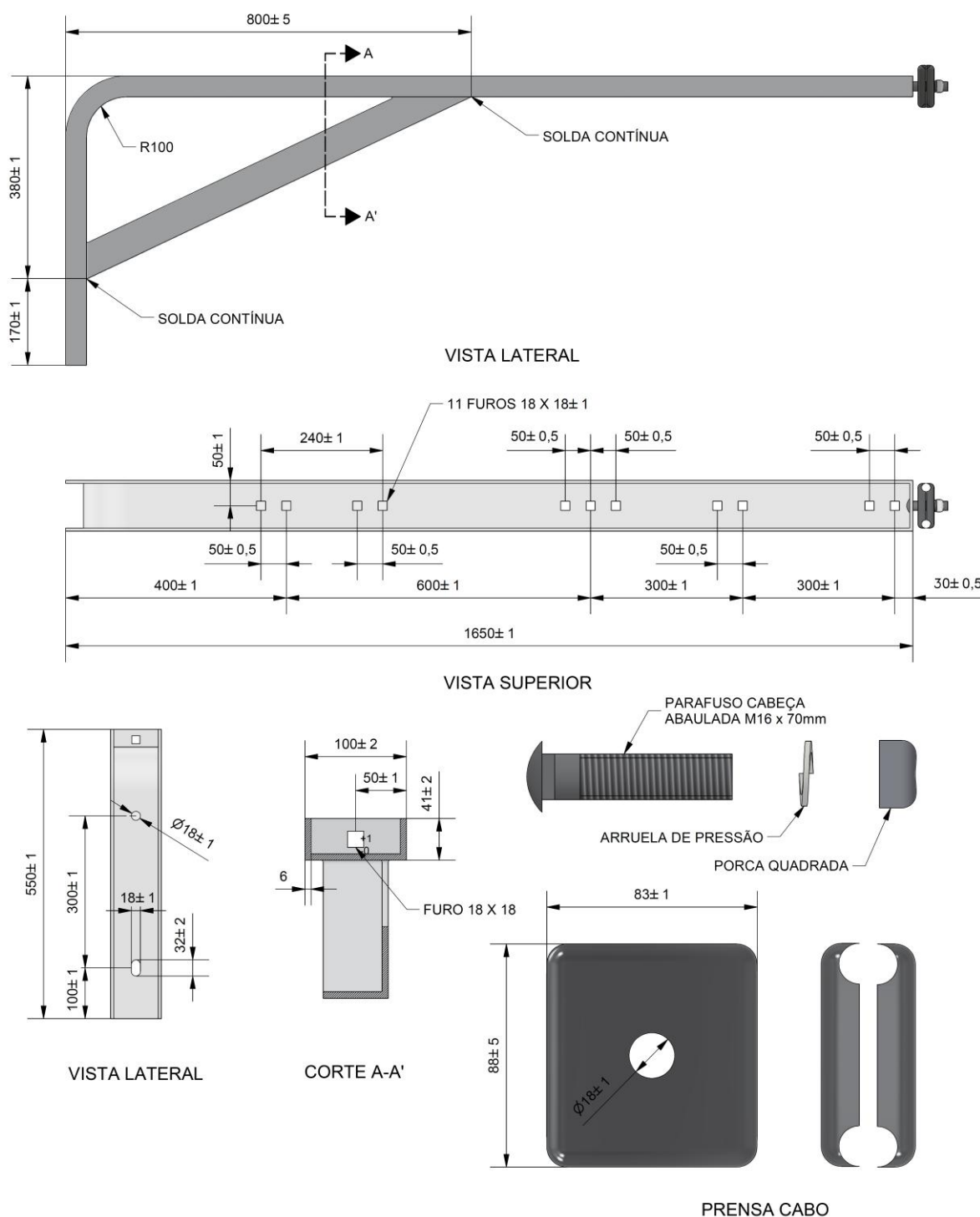
Figura 1 - Braço Afastador Horizontal
